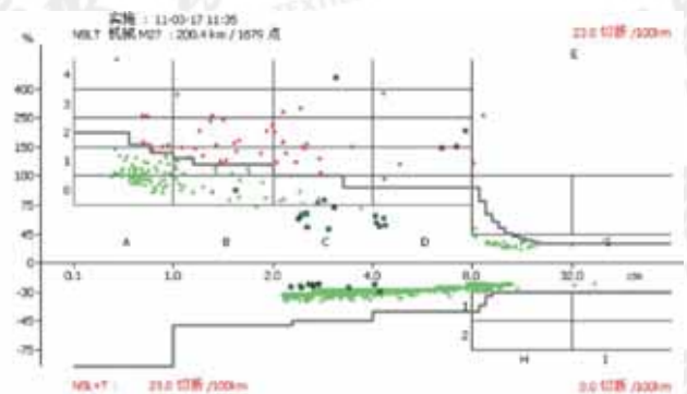
图 2 使用机械搓捻捻接器及优化捻接工艺后的散点图
