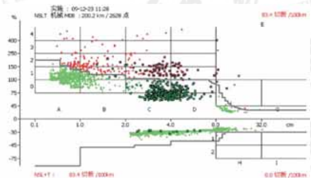
图 1 使用空气捻接器的捻接散点图
